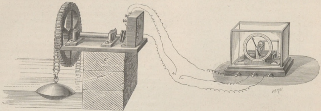
APARATO INDICADOR DEL NIVEL DE AGUA
