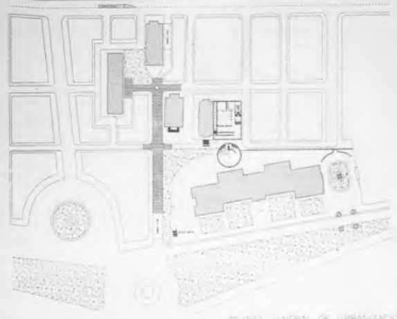
PLANTA GENERAL DE URBANIZACIÓN ESCALA 1/1000
