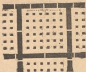
Fig. 119. — Plan de l'Apadâna d'Artaxerxès (d'après Dieulafoy).
