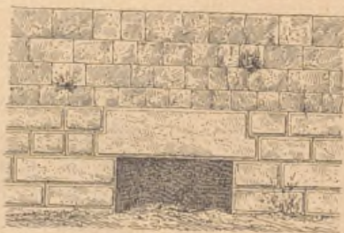
Fig. 166. — La porte occidentale. Etat actuel (d'après M. de Vogüé).
