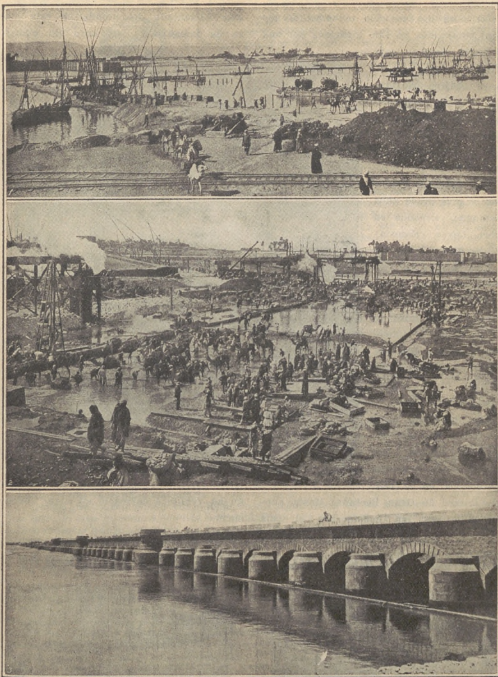
1. Las represas de Esneh que se inauguraron por el Kedive el 9 de Febrero último.—2. Grupo de operarios trabajando.—3. Vista de una parte de las obras
